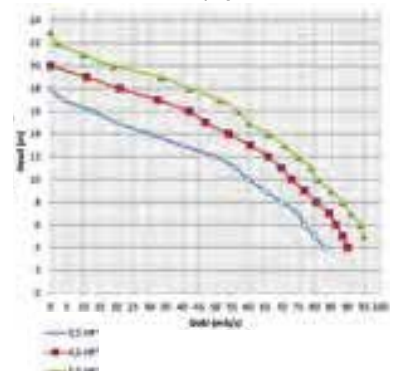
Debi Diyagramı
